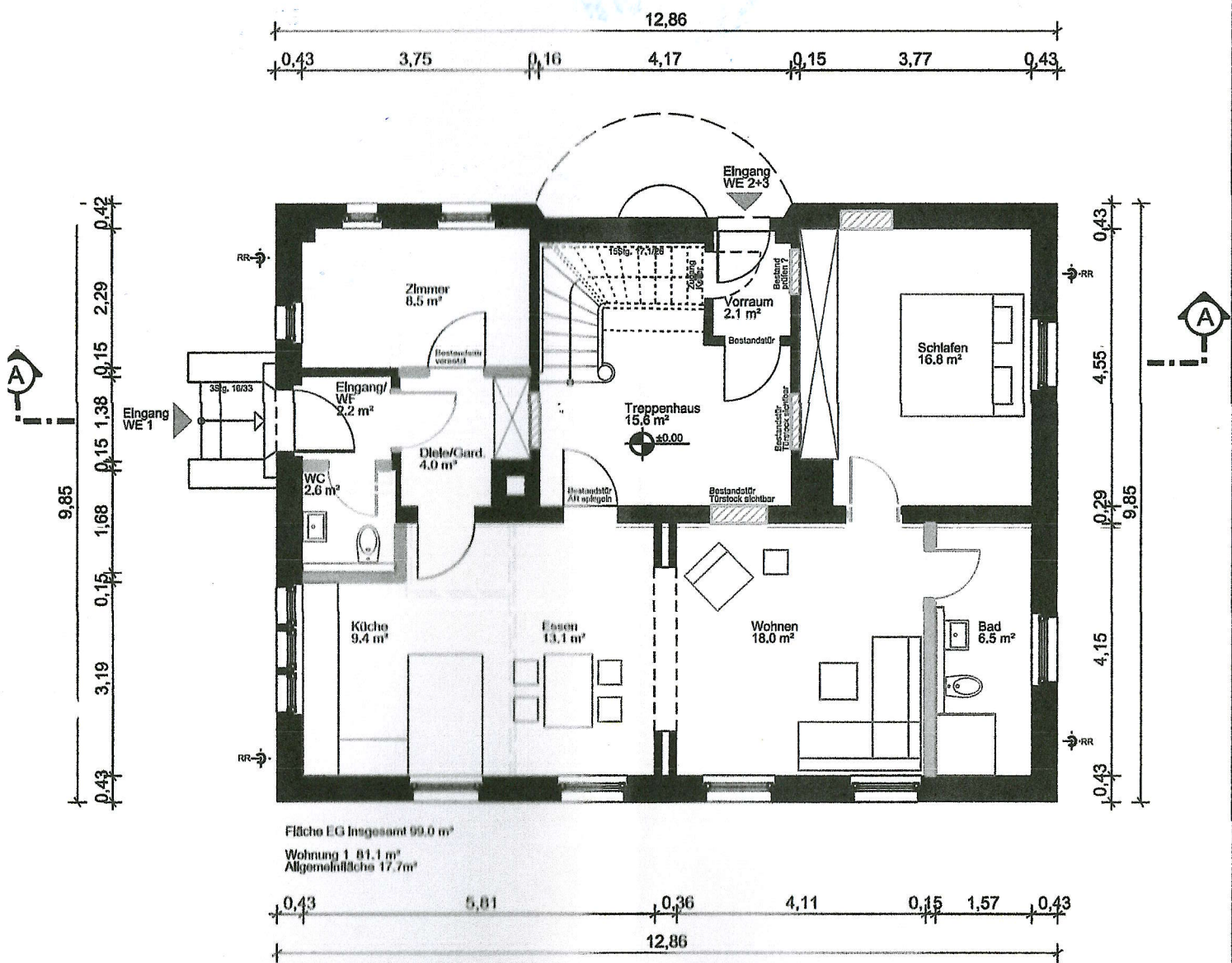
Grundriss Erdgeschoss
