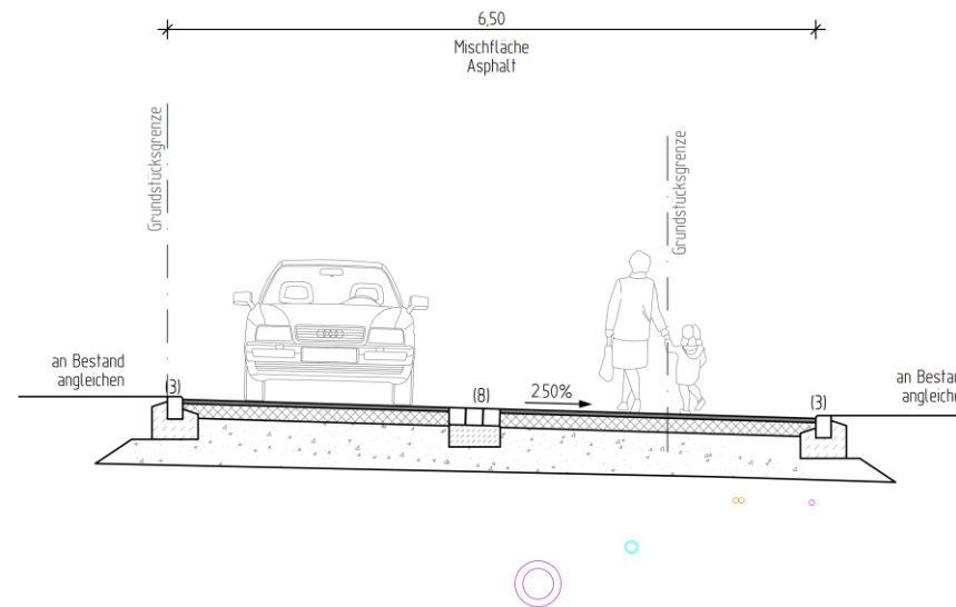
Regelquerschnitt 7 Wendeanlage Gaßbacherweg
