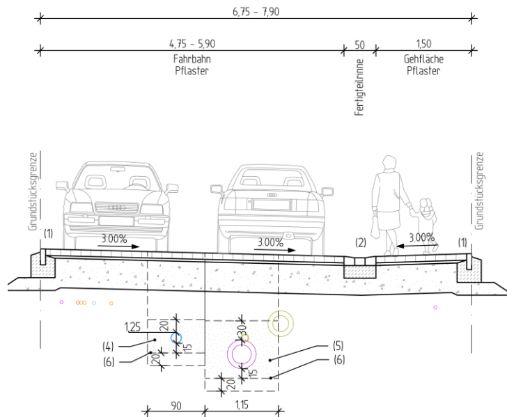
Regelquerschnitt 6: Gaßbacherweg Ost
