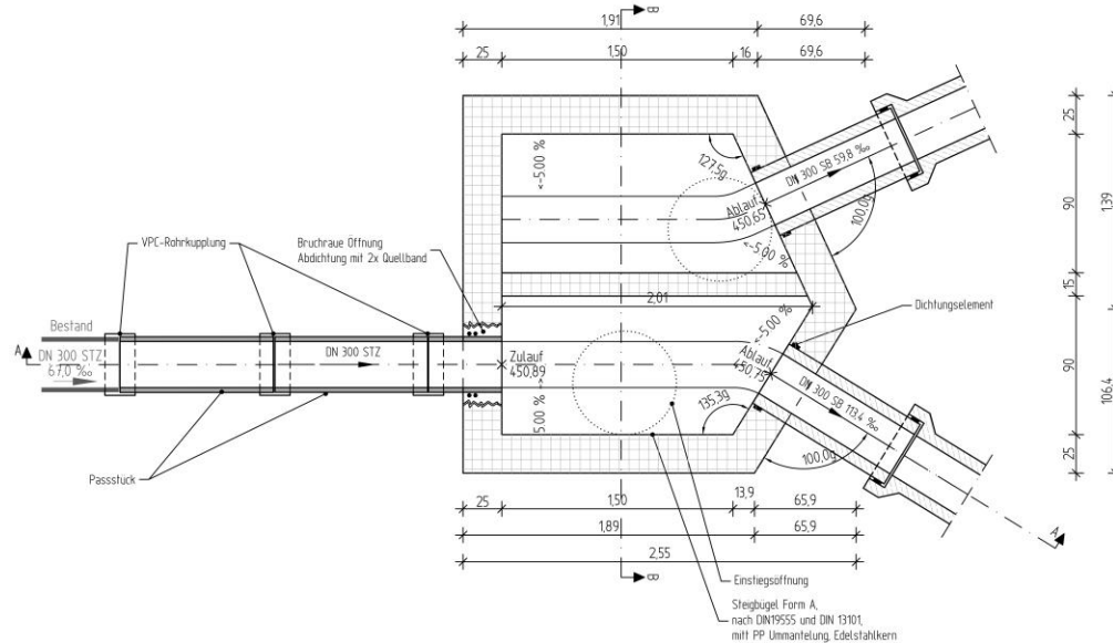
Grundriss
