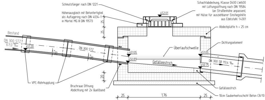
Schnitt A-A
